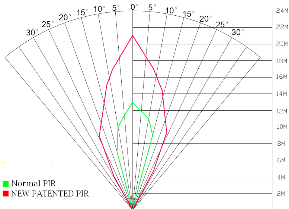
Рис. 7 Сравнение стандартного (зел) и нового (кр) датчиков движения
