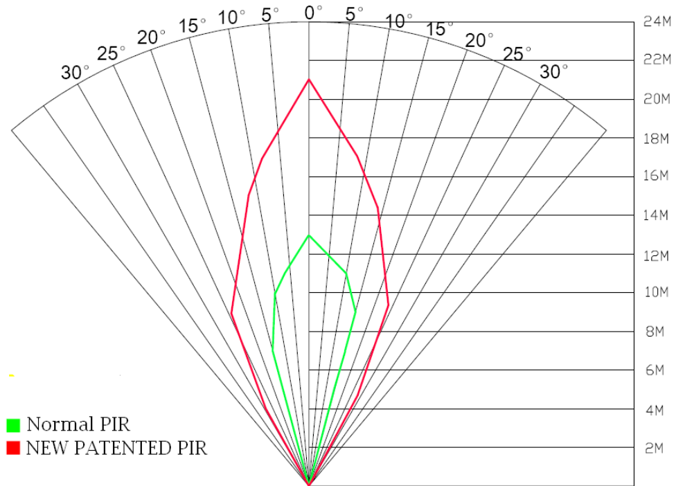
Рис. 7 Сравнение стандартного (зел) и нового (кр) датчиков движения
